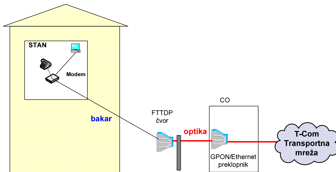
Slika 36. Način realizacije FTTP koncepta u pristupnoj mreži
